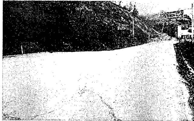
Chunchi; Falla en carpeta y talud inestable
