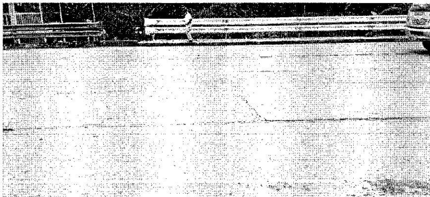
Ilustración 9. Presencia de fisuras longitudinales y transversales en la capa de rodadura (tablero)
