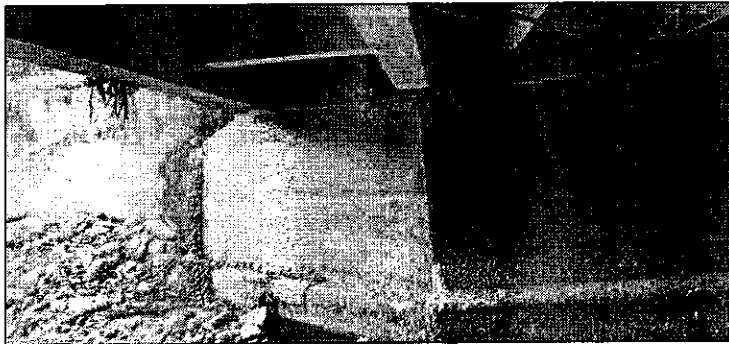
Ilustración 4. Vista frontal Muro de Ala en Estribo (Margen izquierdo - Aguas arriba)
