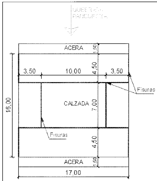
Ilustración 8. (Implantación) Esquema de ubicación de fisuras en la capa de rodadura visibles
