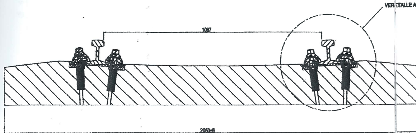
SECCIÓN D-D
