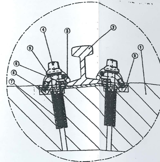
DETALLE A
