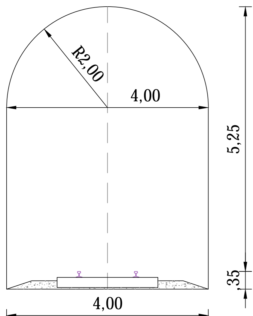
GALIBO TIPICO EN RECTA
