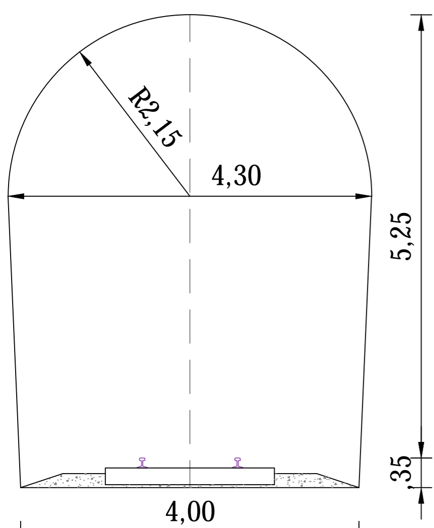
GALIBO TIPICO EN CURVA
